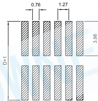
P.C.B Layout
